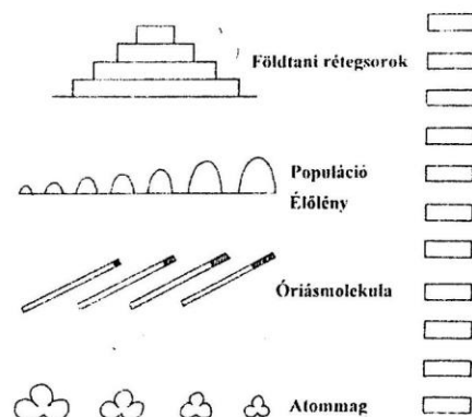
2. ábra. A természeti jelenségek anyagszerkezeti hierarchiája az egymásra rétegződő jelenségszintek oszlopa látható az ábra jobb szélén. Kiemeljük közülük azokat, amelyeken az idő mérésére alkalmas állapot sorokat ismertek föl. Ezek az állapot sorok alkotják magukat a változást értelmező órákat az egyes leírt szinteken. A változások sorozatának fölismerése az egyes szinteken a következő évszázadokban történtek. Legfölülről kezdve: Földtani rétegsorok (Steno nyomán) - 18. század. Az élővilág evolúciója (Darwin) - 19. század. Óriásmolekulák genetikai órája - 20. század második fele. Atommagok bomlása - 20. század első fele.
